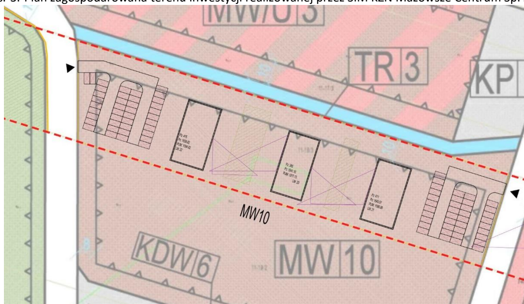
Rys. 3. Plan zagospodarowania terenu inwestycji realizowanej przez SIM KZN Mazowsze Centrum Sp. z o.o.
